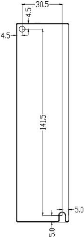
图 2-1 CL3C-EC808AC 安装尺寸图(单位：mm) ※ 设计安装尺寸时，注意考虑端子大小及布线！
