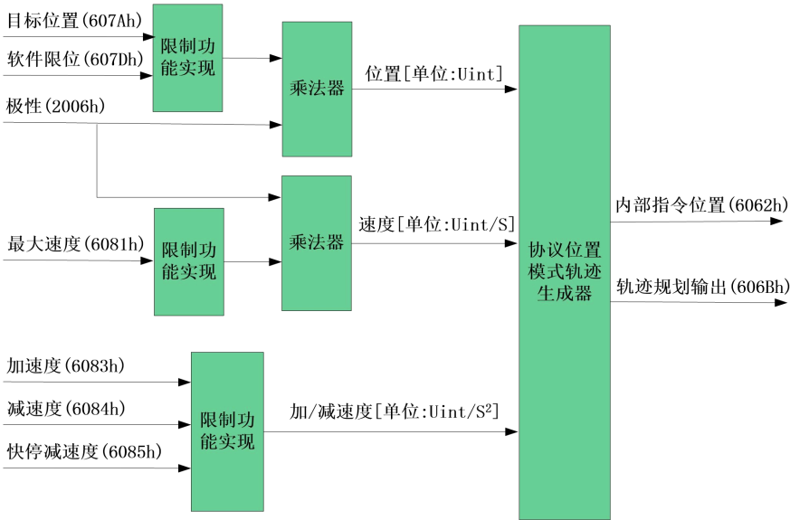
图 7.8PP 模式的轨迹生成
