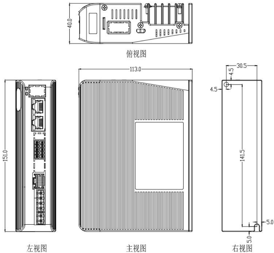
图 2-1 CL3C-EC808AC 安装尺寸图(单位：mm) ※ 设计安装尺寸时，注意考虑端子大小及布线！
